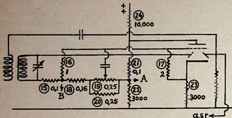
De omcirkelde getallen zijn aanwijzingen uit het origineele fabrieksschema.
