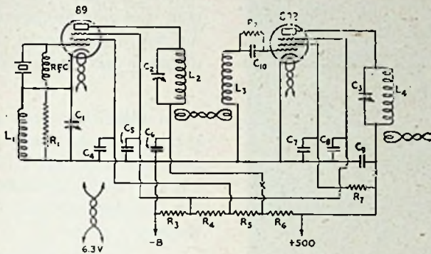
Fig. 4. Principeschema van den 10 meter-zender, waarin 2 lampen 2 maal verdubbelen.
